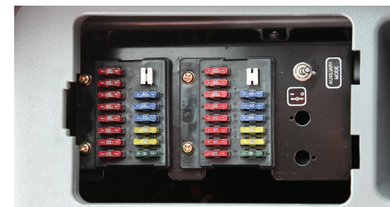
Cómoda caja de fusibles La caja de fusibles se encuentra en el compartimento de almacenamiento junto al asiento, en un ámbito despejado y de fácil acceso.
